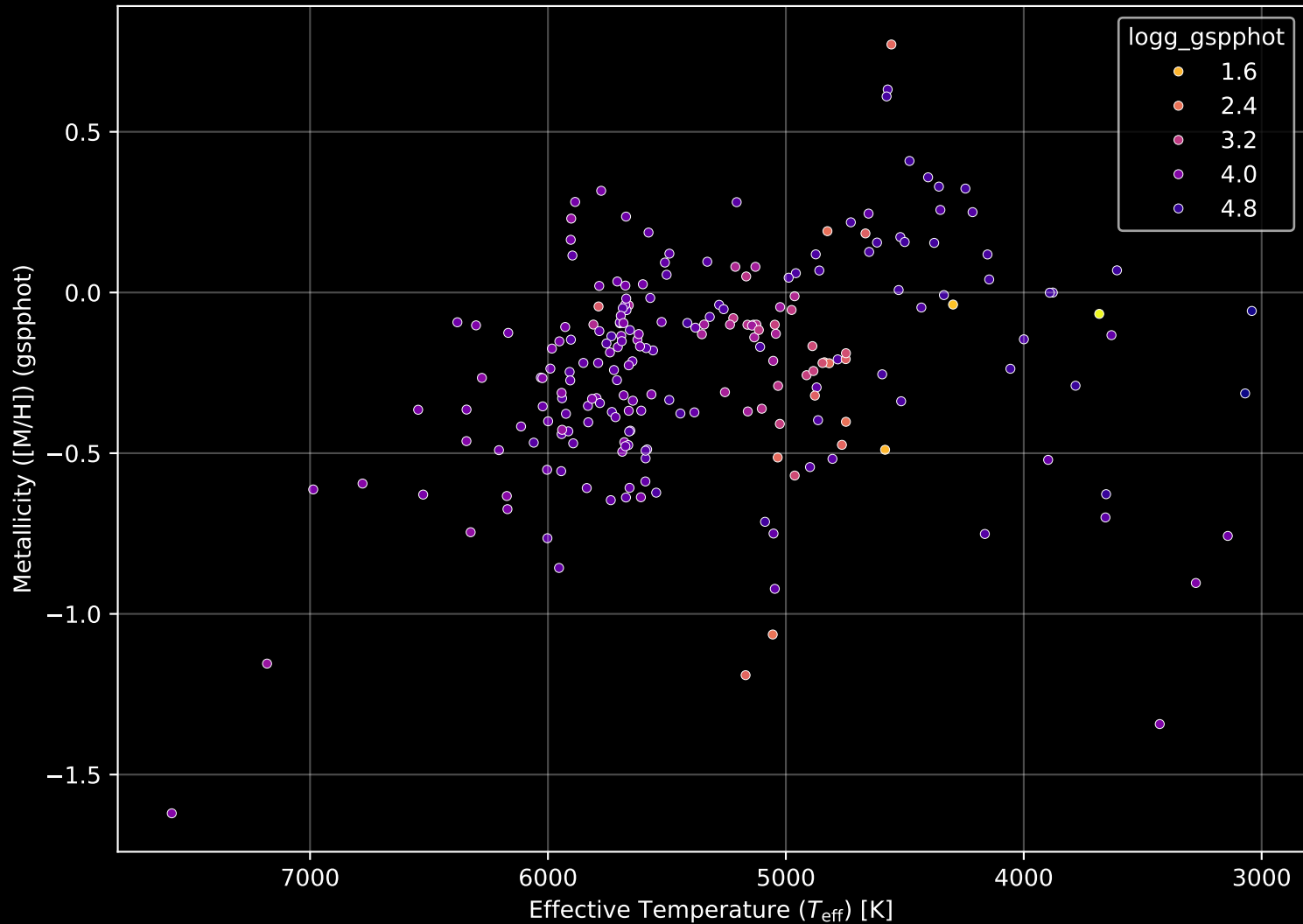
APOGEE DR17 Field: [167-55] Stellar Population Parameters (n= 220)
